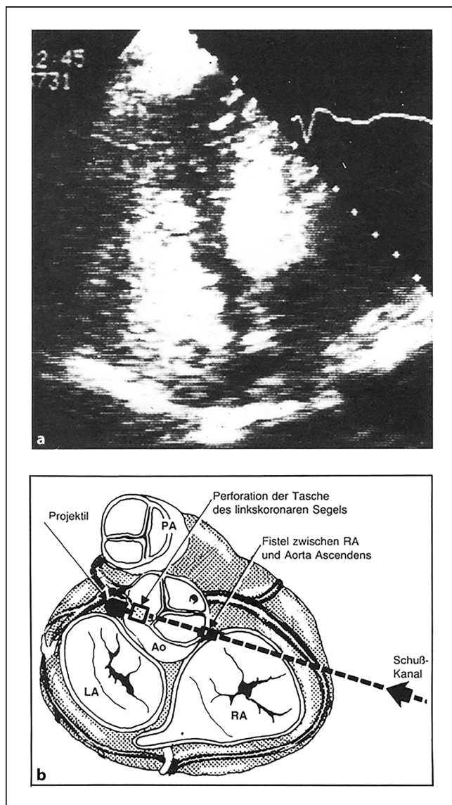
Abb. 1 ◀ a 4-Kammer-Blick vor Injektion des Kontrastmittels in die Aortenwurzel (Ao), nach Injektion intensive Kontrastierung des rechten Vorhofs (RA) und rechten Ventrikels. b Rekonstruktion des Schusskanals, LA linker Vorhof, PA Pulmonalarterie. (Aus [8]; mit freundlicher Genehmigung von © 1984 Richard Pflaum Verlag GmbH & Co. KG. All Rights Reserved)
